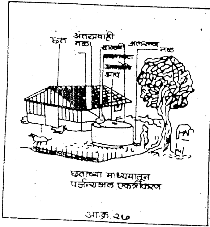
छतावरील पर्जन्यजल साठवणीसाठी रचना
