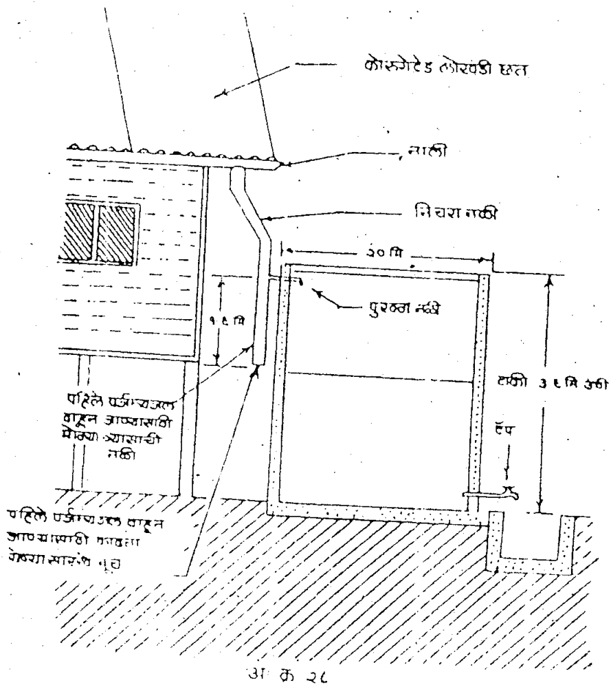
छतावरील पर्जन्यजल साठवणीसाठी रचना
